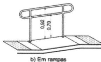
b) Em rampas Altura dos corrimãos em rampas e escadas
