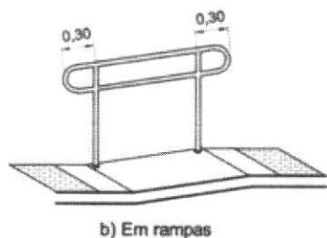
b) Em rampas - Prolongamento do corrimão -
